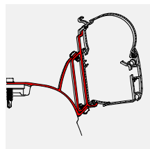
Multivan adaptér
