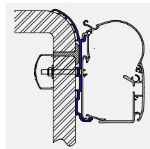
Bürstner zahnutý
