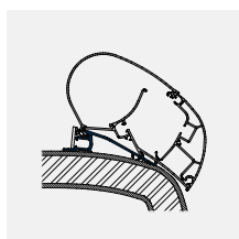
Hymer SX
