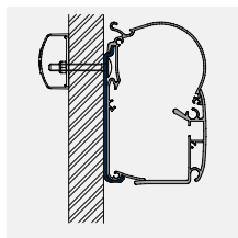
Plochý adaptér
