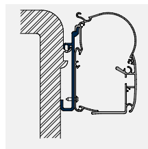
Rapido 2007, 8, 9
